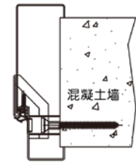
可调节框 MultiFrame 框中孔螺钉安装
