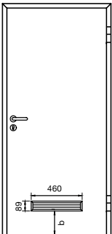
尼龙百页 (适用于门型 ZK-, HT, HT40)
