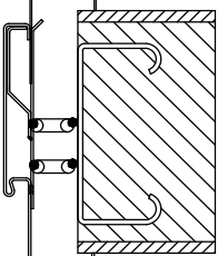
可调节框 VarioFrame 预埋件焊接 D1 型
