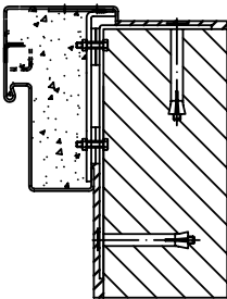
反侧角框连接
