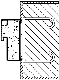
预埋件焊接 D1 型
