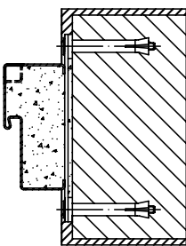
框外拉板 B 型
