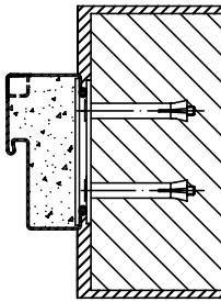
外加预埋件焊接 D2 型
