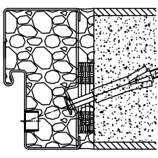
框中孔 A1 型
