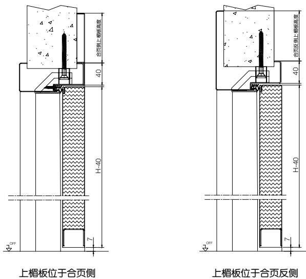
多功能可调节框 MultiFrame 配单层上楣板截面图
