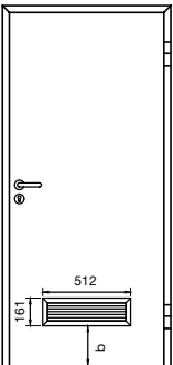
钢质百页 (适用于门型 ZK-)
