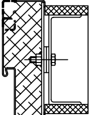
石膏板龙骨 / 钢结构 F 型
