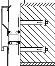
可调节框 VarioFrame 外加预埋件焊接 D2 型
