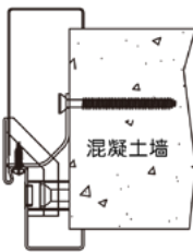
可调节框 MultiFrame 拉板连接 G 型
