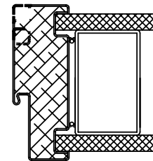
石膏板龙骨 / 钢结构 E 型
