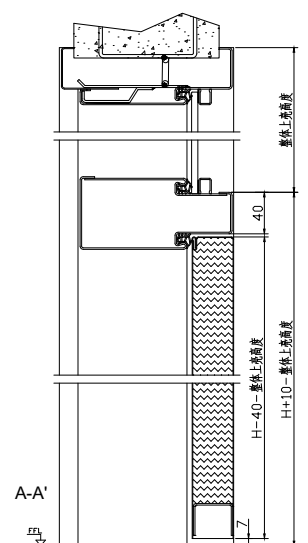
可调节框 VarioFrame配整体上亮截面图
